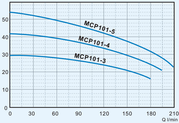
H m PERFORMANCE CHART AT n=2900r/min 折算到2900r/min时性能
